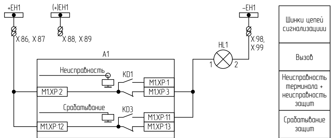
Цепи сигнализации
