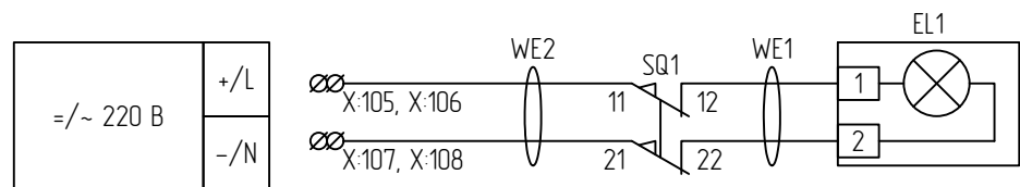
Цепи освещения шкафа
