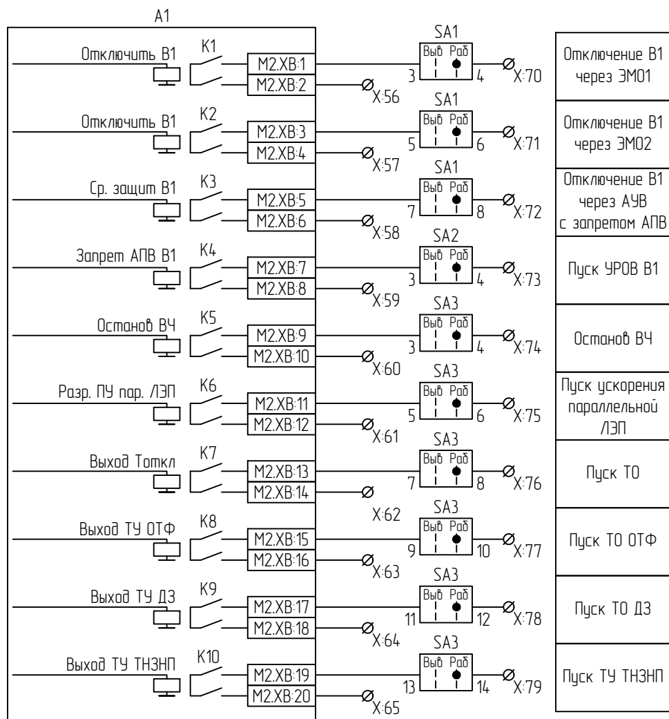
Выходные цепи
